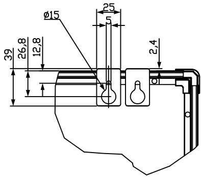
壁掛金具寸法（参考図）
