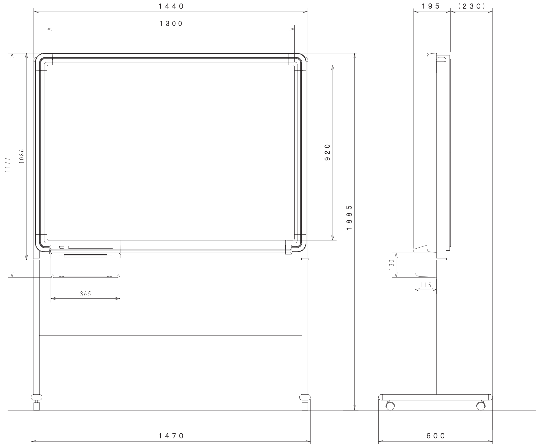
BF-041S 外觀圖
