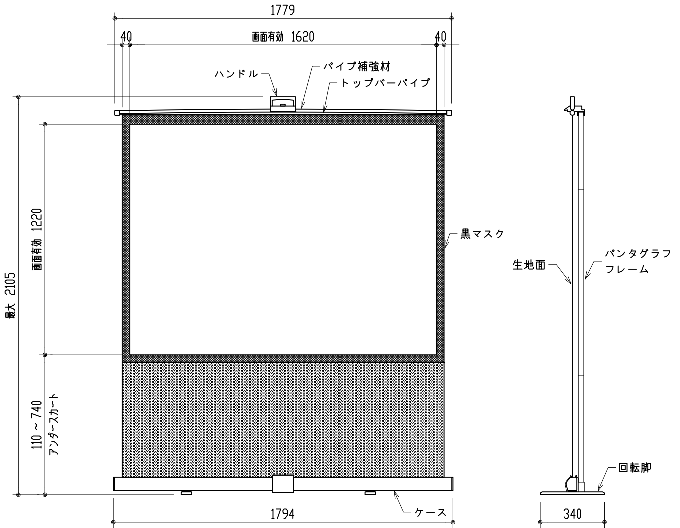
スクリーン設置図 S=1/20
