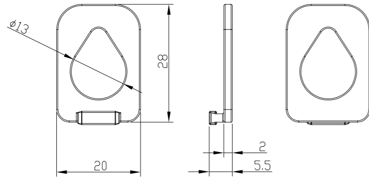
吊り具拡大図
