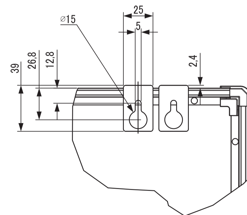
壁掛金具寸法(参考図)
