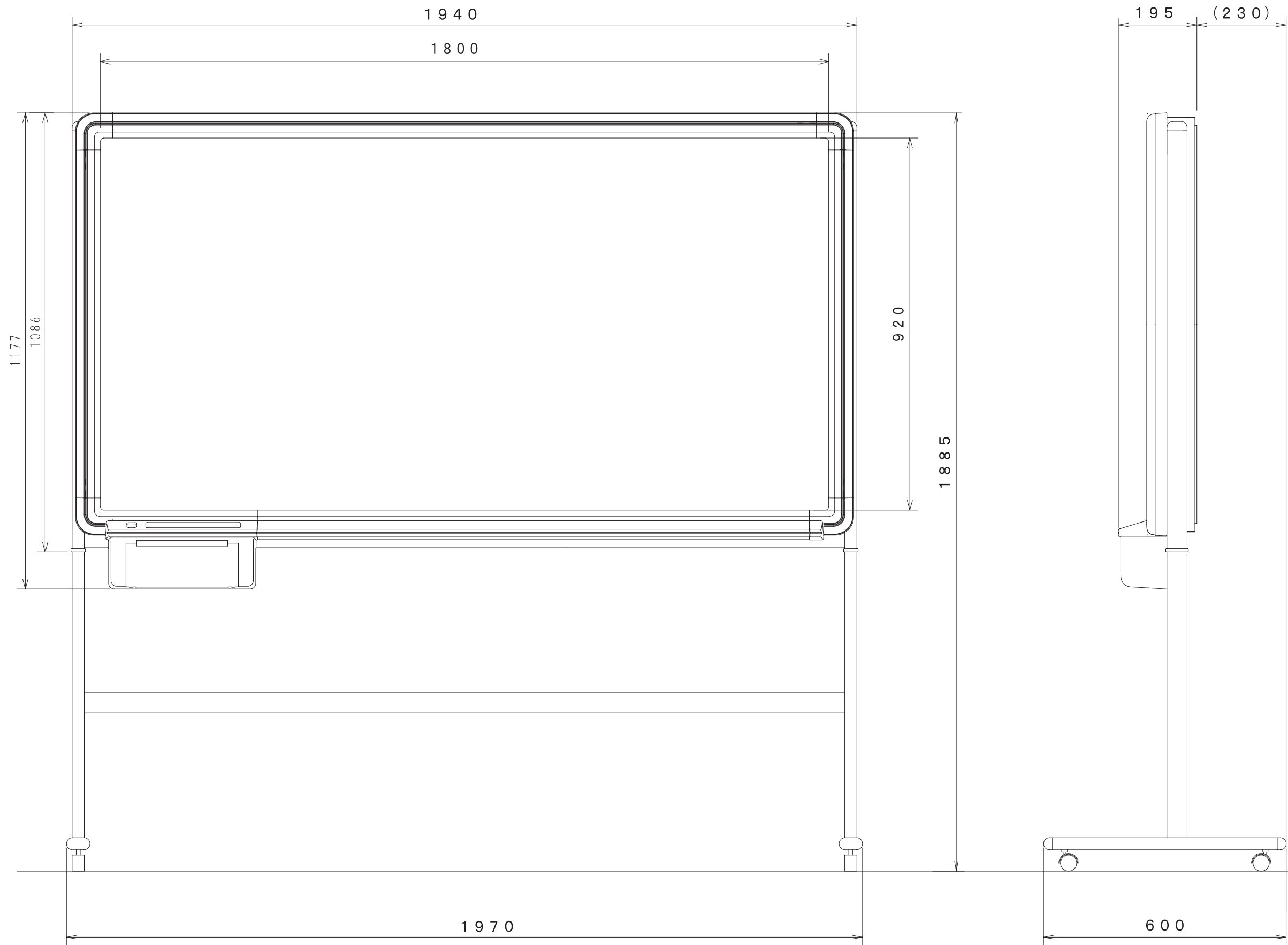
BF-041W 外觀圖
