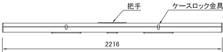
スクリーン収納時ケース外寸 S=1/20
