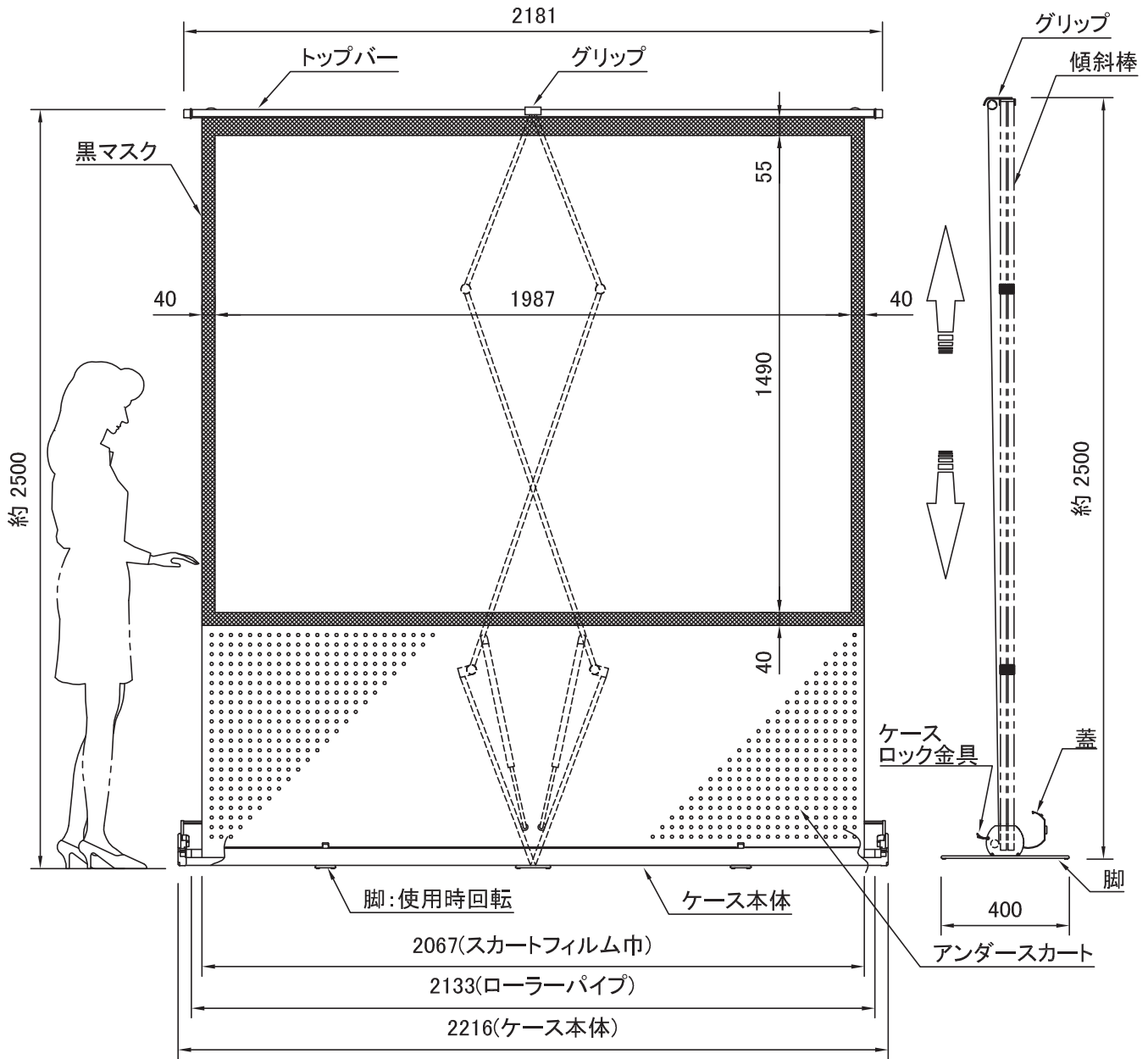
スクリーン設置図 S=1/20
