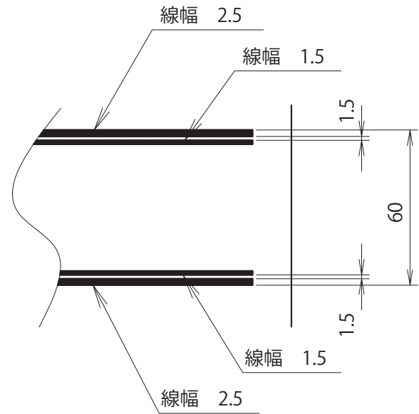
A部野線パターン (1:2)
