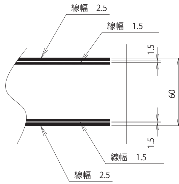
A部罫線パターン (1:2)
